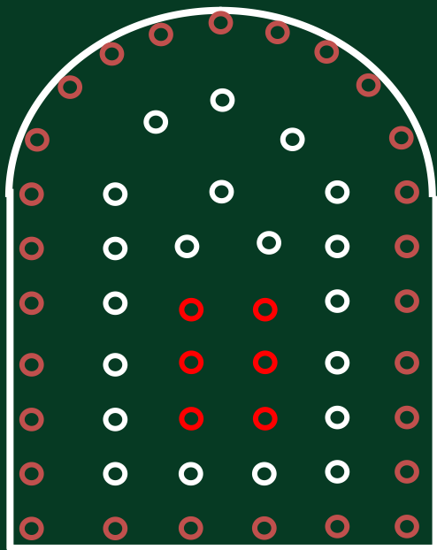
图5-1 炮眼布置图
