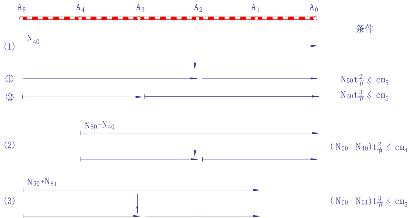
图2-3-20 切割示意图
