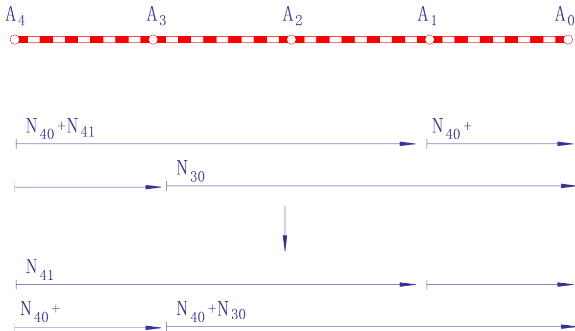
图2-3-19 调流示意图
