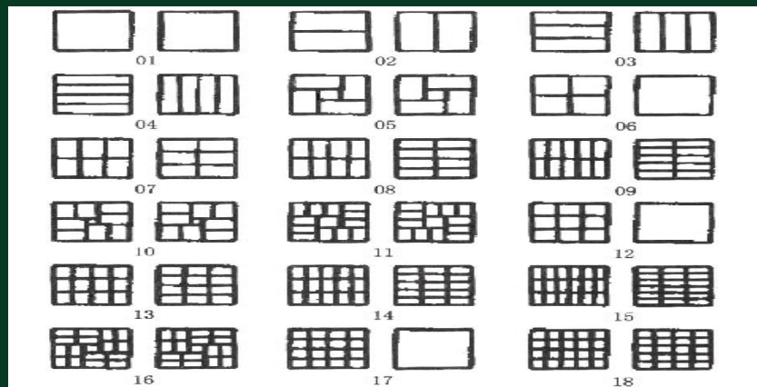
硬质直方体在1140mm×1140mm托盘上的堆码图谱
