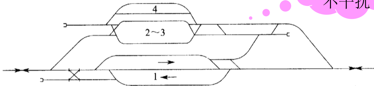
图 3-2 有贯通式货场的横列式货运站
