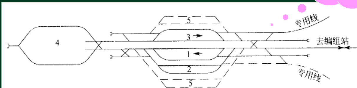
图 3-4 有贯通式货场的纵列式货运站
